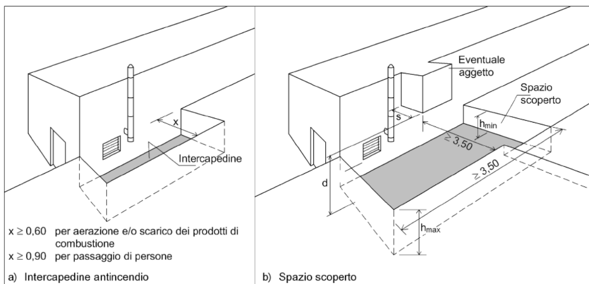
Figura 81.6 - Intercompedine antincendio e spazio scoperto secondo il D.M. 30 novembre 1983
