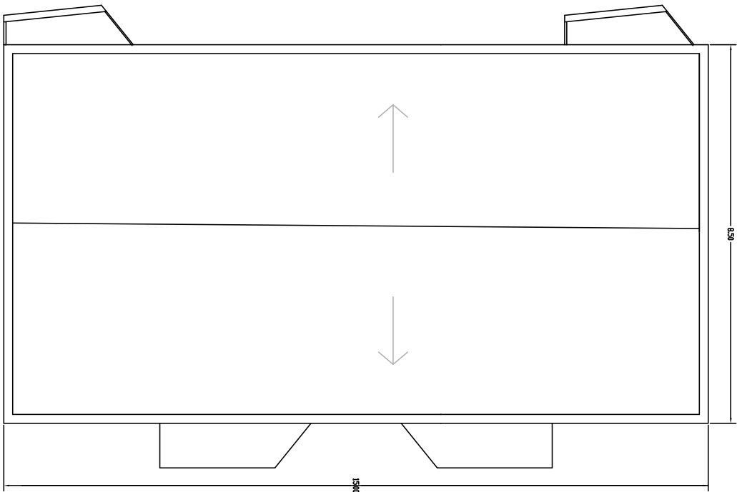
pianta copertura
